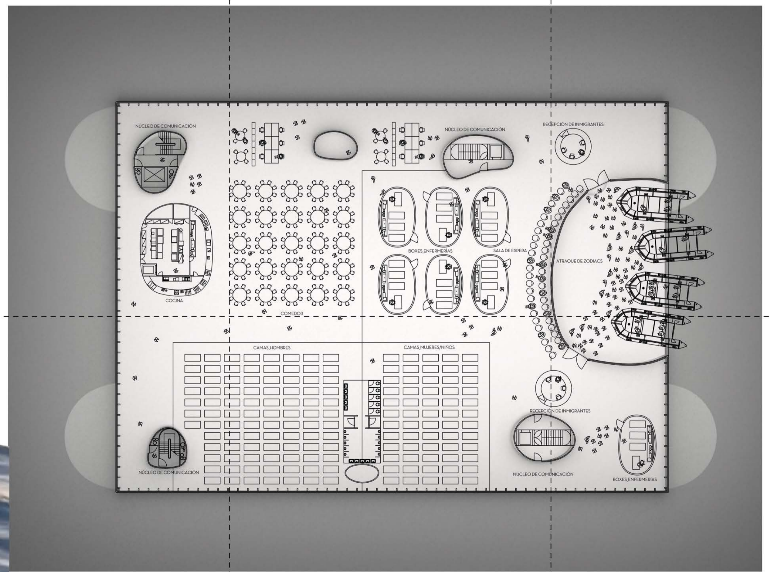
>>Planta de Cuidados de Refugiados+Ataque de Zodiacs+Distribución<Escala1/300<<
