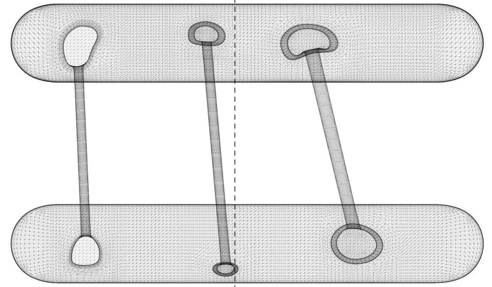
>>Planta de Pantoon//Parte sumergida de la plataforma<Escala1/400<<
