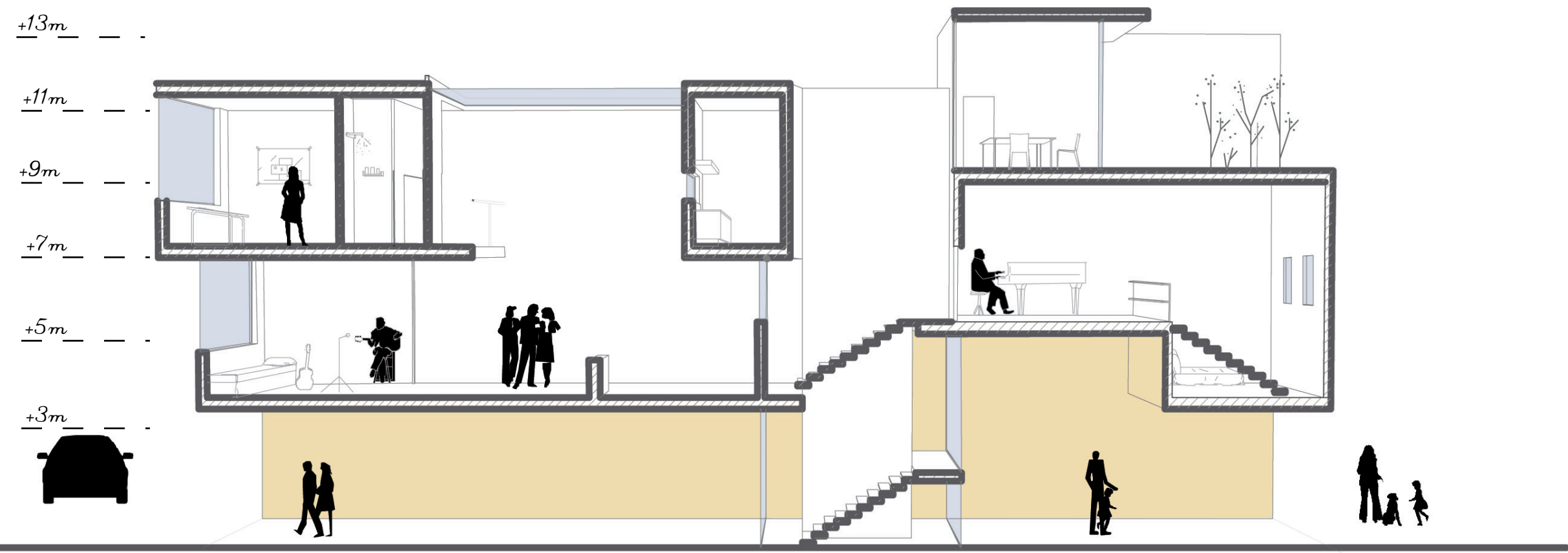
Seccion B-B
