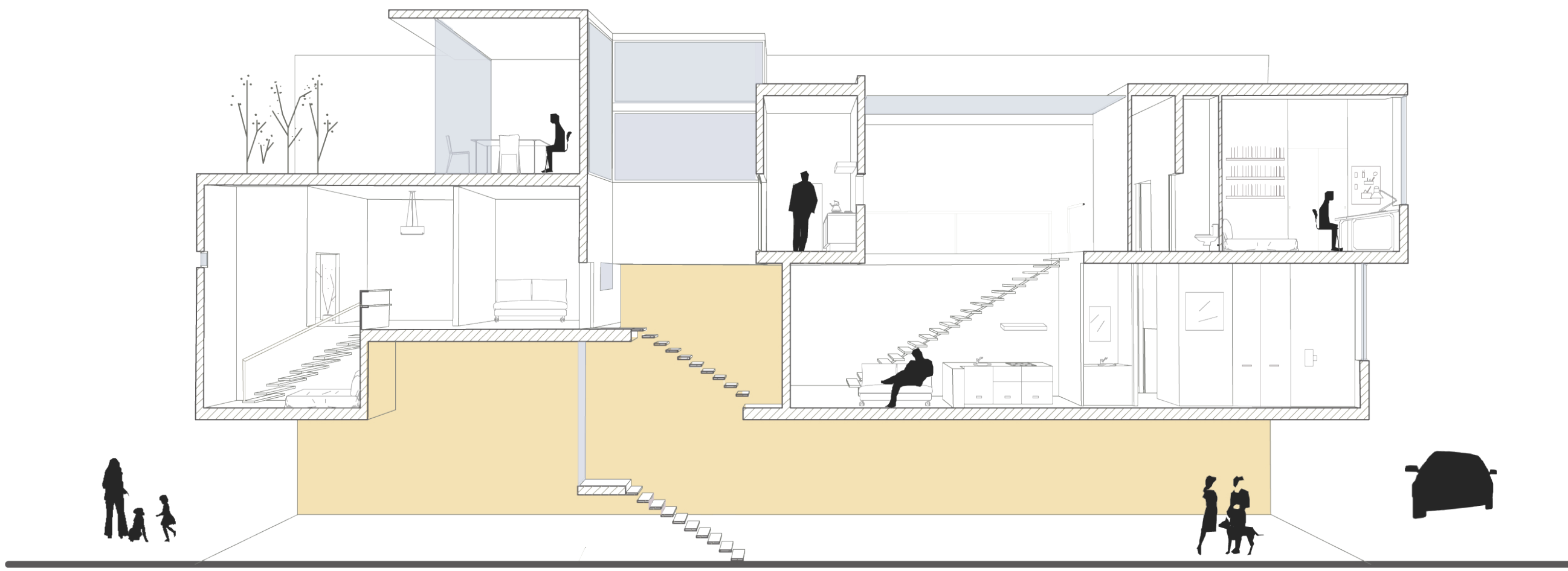
Seccion A-A
