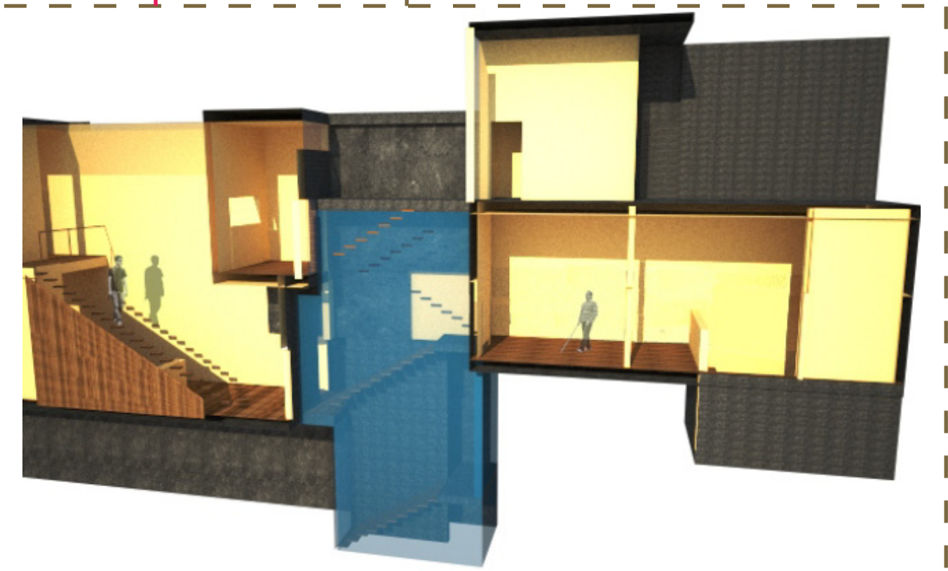
Seccion B-B
