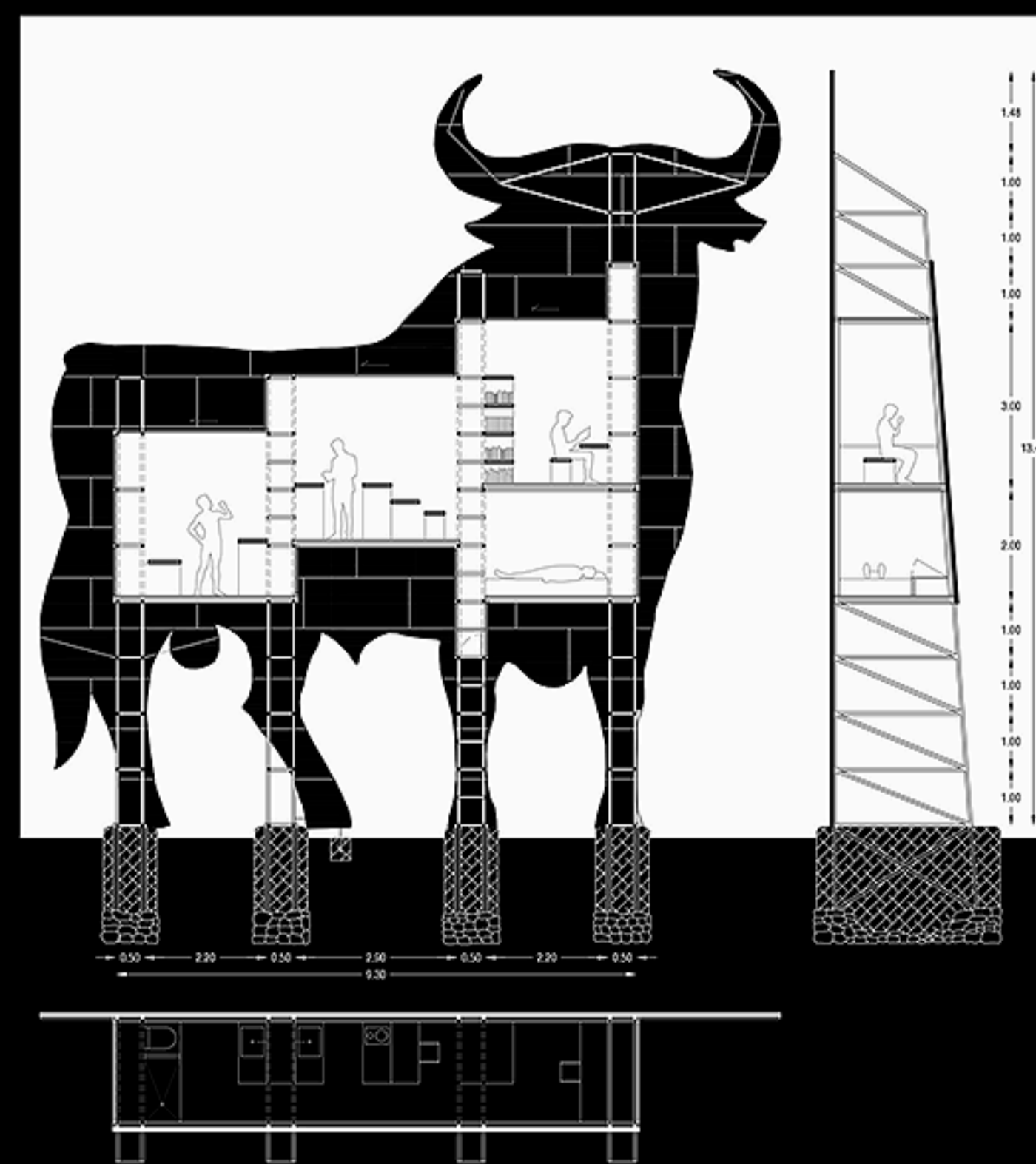
▲ Planta alzado y sección de la propuesta _ e 1:100
