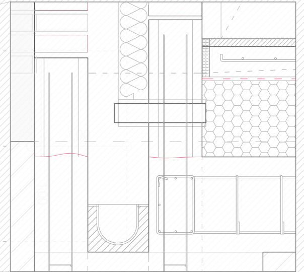
detalle de cámara y encuentro con el terreno! {E1:10}
