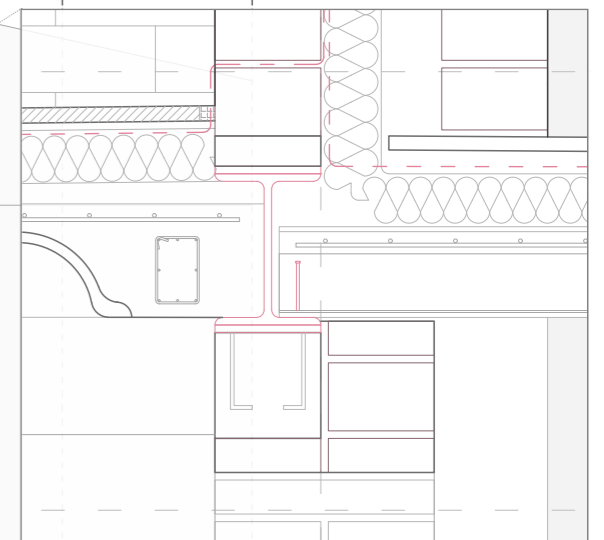
detalle del paso de forjado cerámica-chapa! {E1:10}
