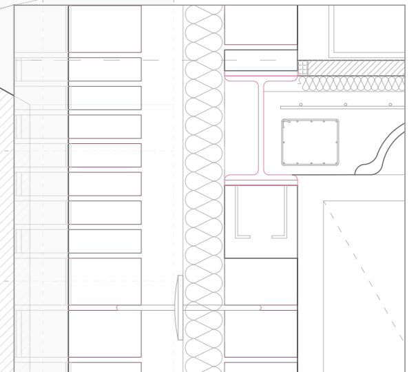
detalle de la solución para la fachada! {E1:10}
