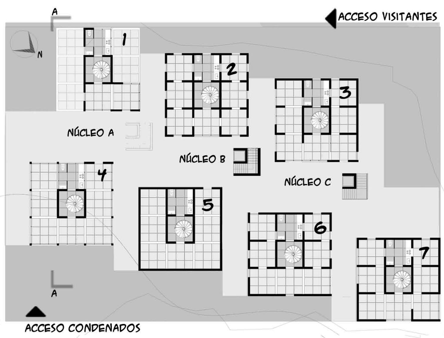
PLANTA COMÚN-NÚCLEOS HÚMEPOS Y ZONA DE "ESPARCIMIENTO"
