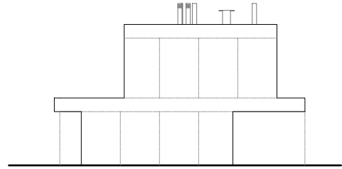
ALZADO NORTE
