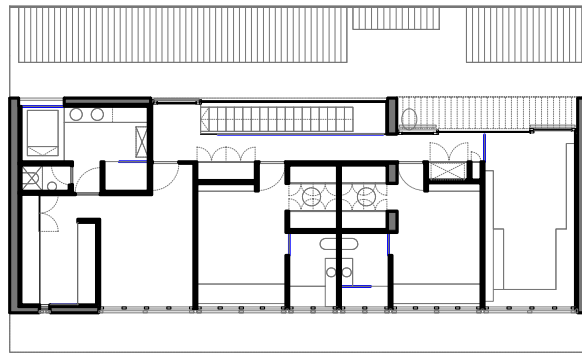
PLANTA PRIMERA
