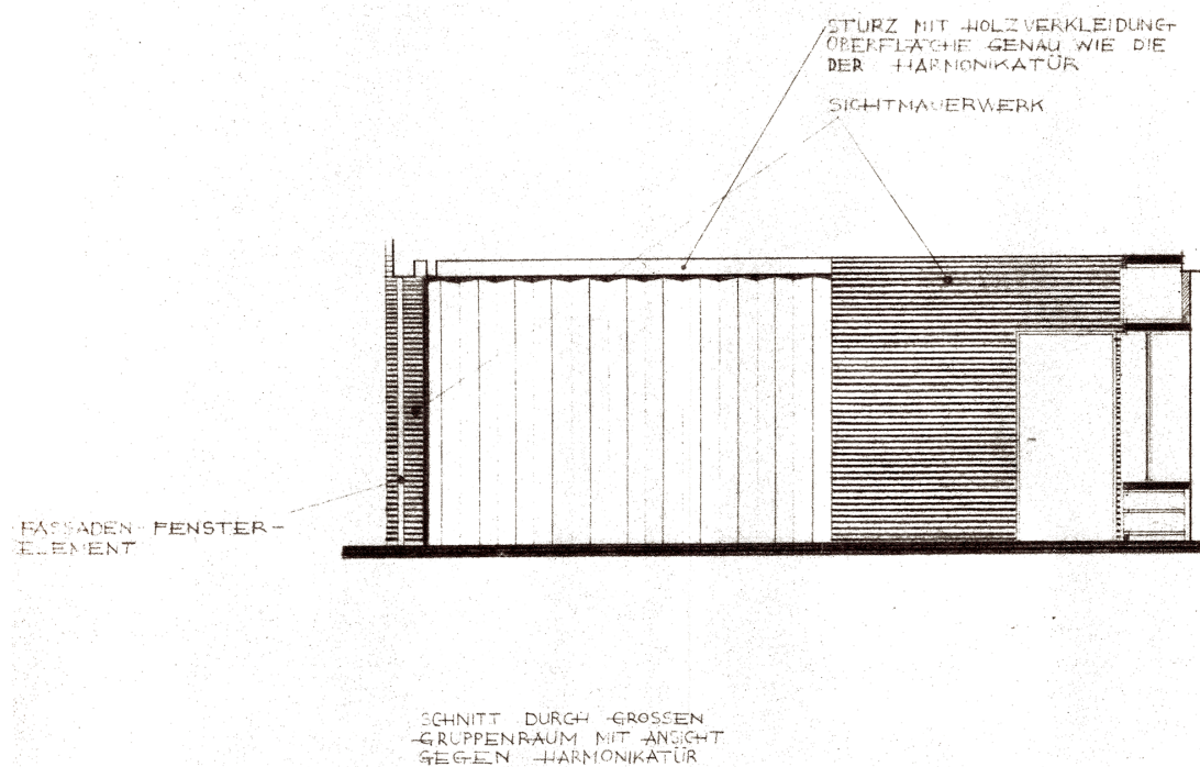
Figura 11. Sección por dentro del aula mostrando en encuentro entre el paramento vertical de ladrillo cara vista y la Harmonikatür. Navarro, Pablo.1960
