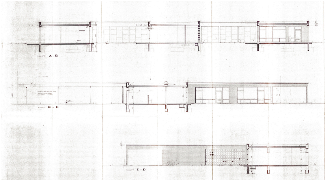
Figura 8. Secciones del proyecto por la zona del Kindergarten. Navarro, Pablo. 1959.
