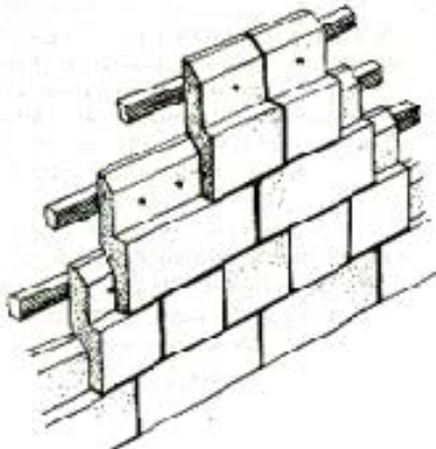
Figura 1. Esquema de paneles de ladrillo a cara vista.
