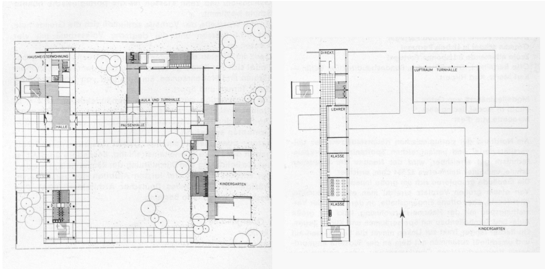
Figura 5. Anteproyecto del conjunto del Colegio Alemán de Valencia, planta baja y planta tipo. Meyer F.S. 1960, 599.
