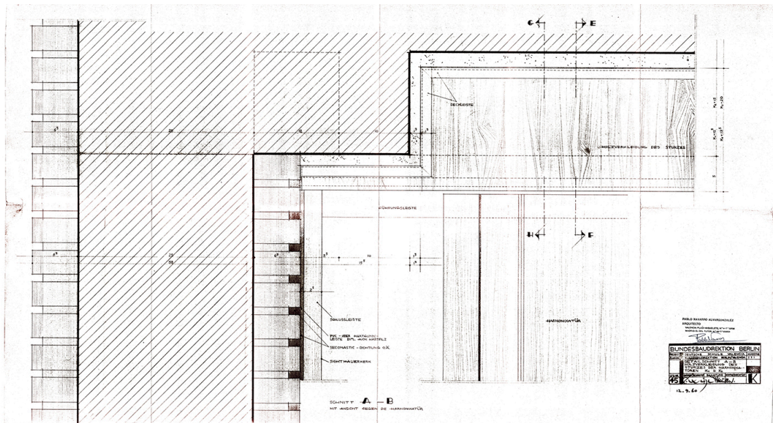
Figura 12. Detalle constructivo de la esquina superior izquierda de la figura 12, del encuentro entre pilar, viga y Harmonikatür. Navarro, Pablo.1960
