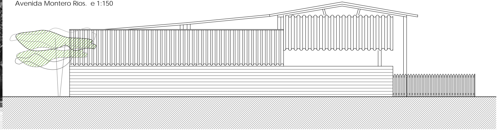
ESTADO ACTUAL. ALZADO SUR. Avenida Montero Ríos. e 1:150
