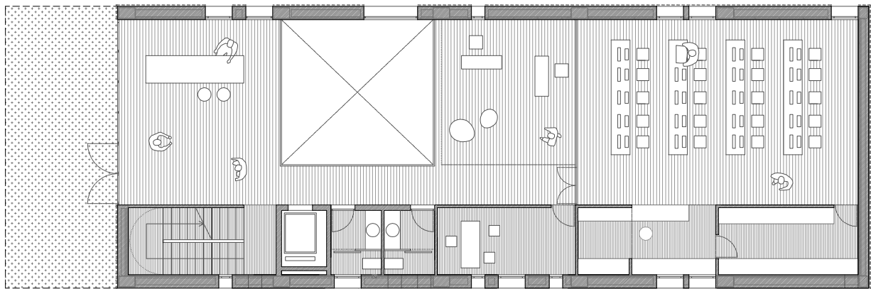
planta acceso cota +/-0,00 m
