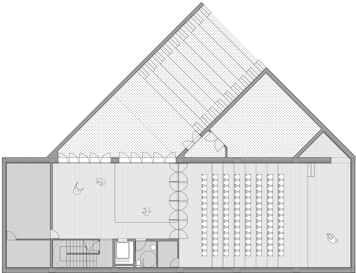
planta sótano cota -3,40 m
