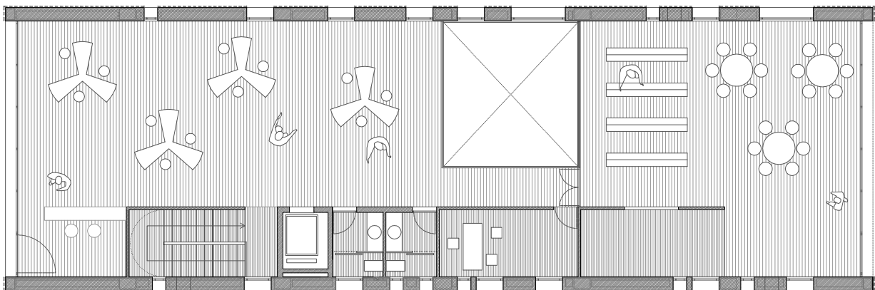
planta primera cota +3,74 m
