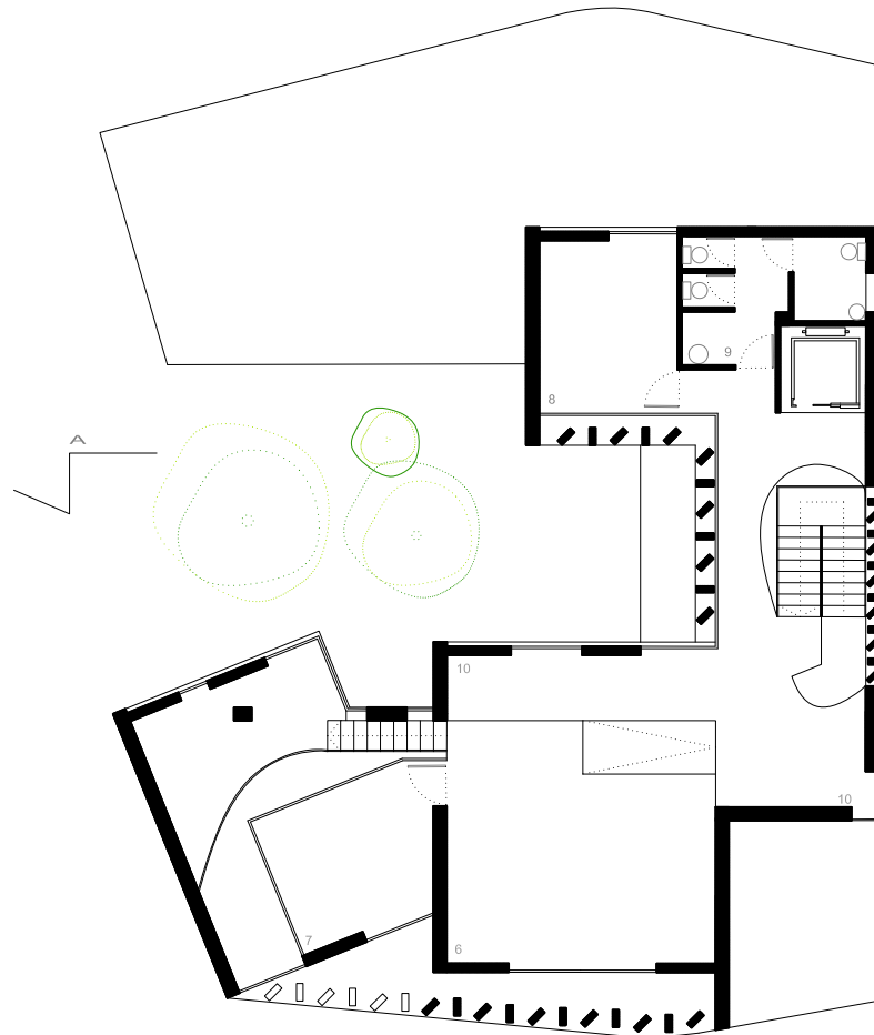
PLANTA PRIMERA
