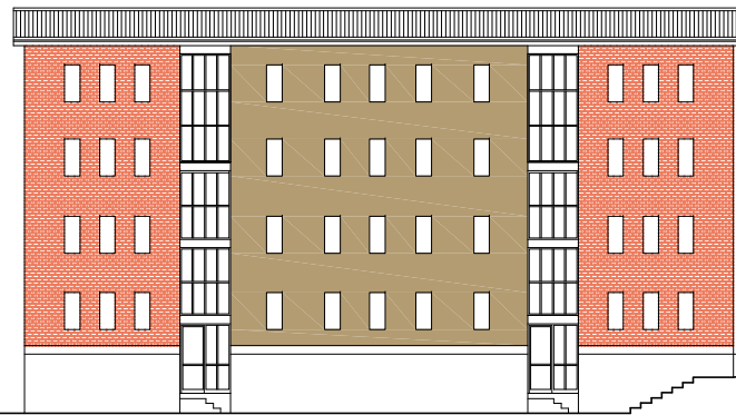
AI-2. ALÇAT INTERIOR 2, PLAÇETA. E: 1/300 EDIFICI 3
