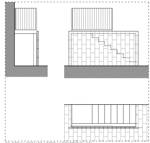
D2. DETALL ESCALES ACCES HABITATGES, E:1/100
