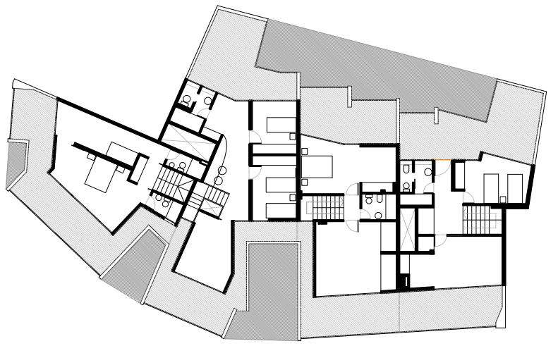
PLANTA BAJO CUBIERTA
