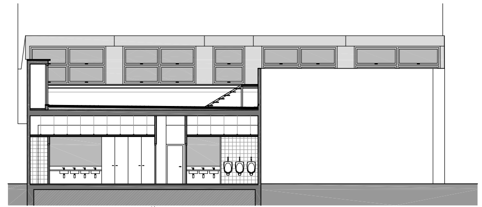
S-9, SECCIO TRANSVERSAL, E: 1/200
