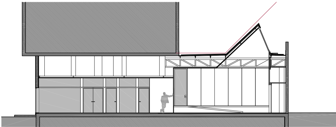
S-6, SECCIO LONGITUDINAL, E: 1/200
