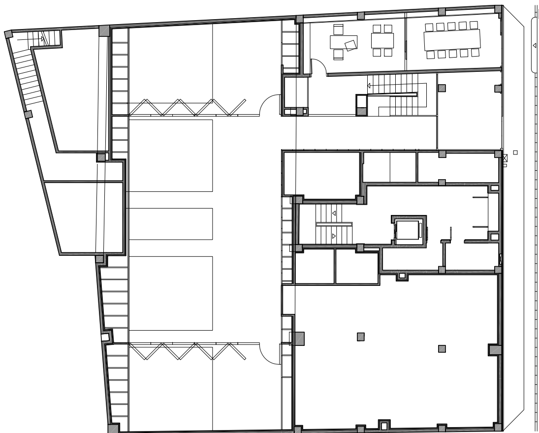
PLANTA ALTELL, E: 1/200
