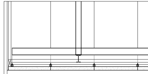
D5, DETALL 5, E: 1/30
