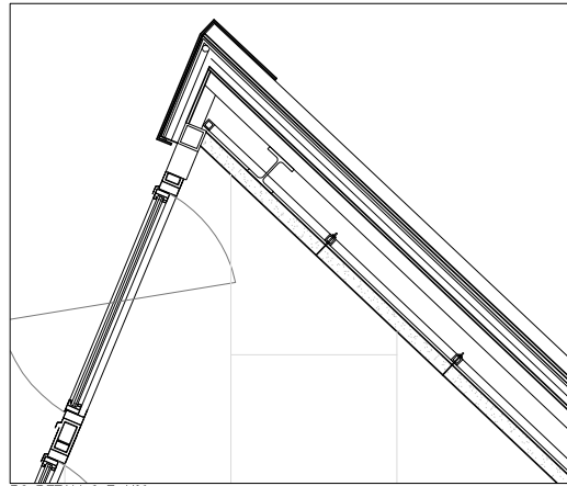
D2, DETALL 2, E: 1/30
