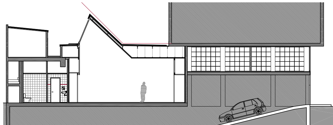
S-2, SECCIO LONGITUDINAL, E: 1/200
