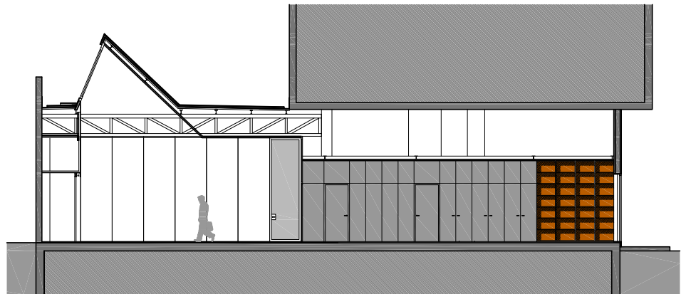
S-1, SECCIÓ LONGITUDINAL, E: 1/200
