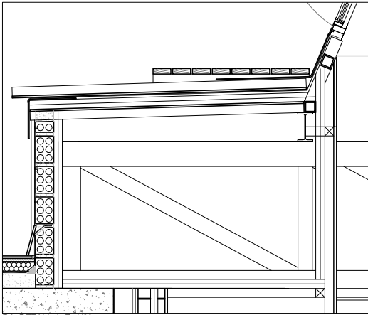
D1, DETALL 1, E: 1/30
