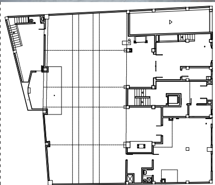
PLANTA BAIXA ESTAT ANTERIOR, E: 1/500
