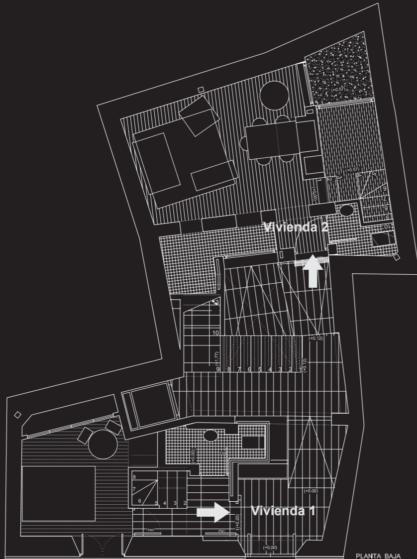
PLANTA BAJA
