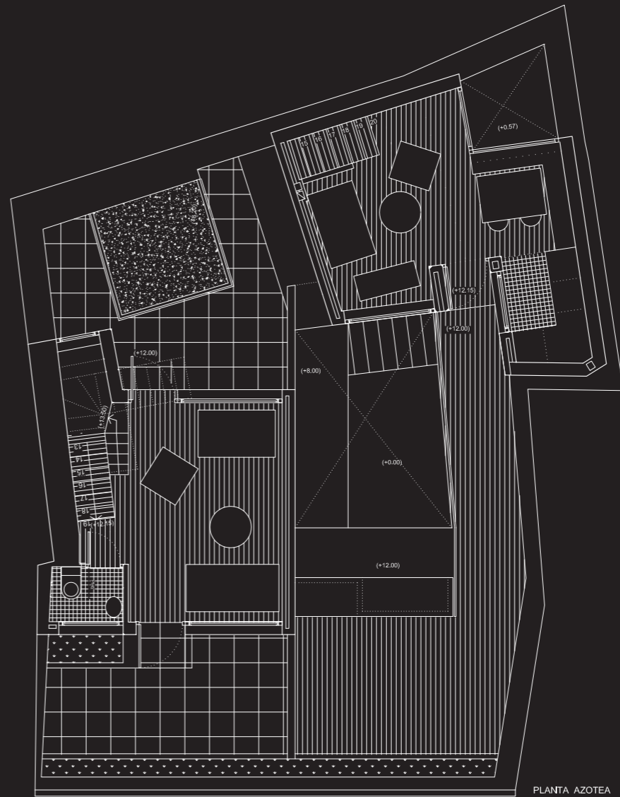
PLANTA AZOTEA
