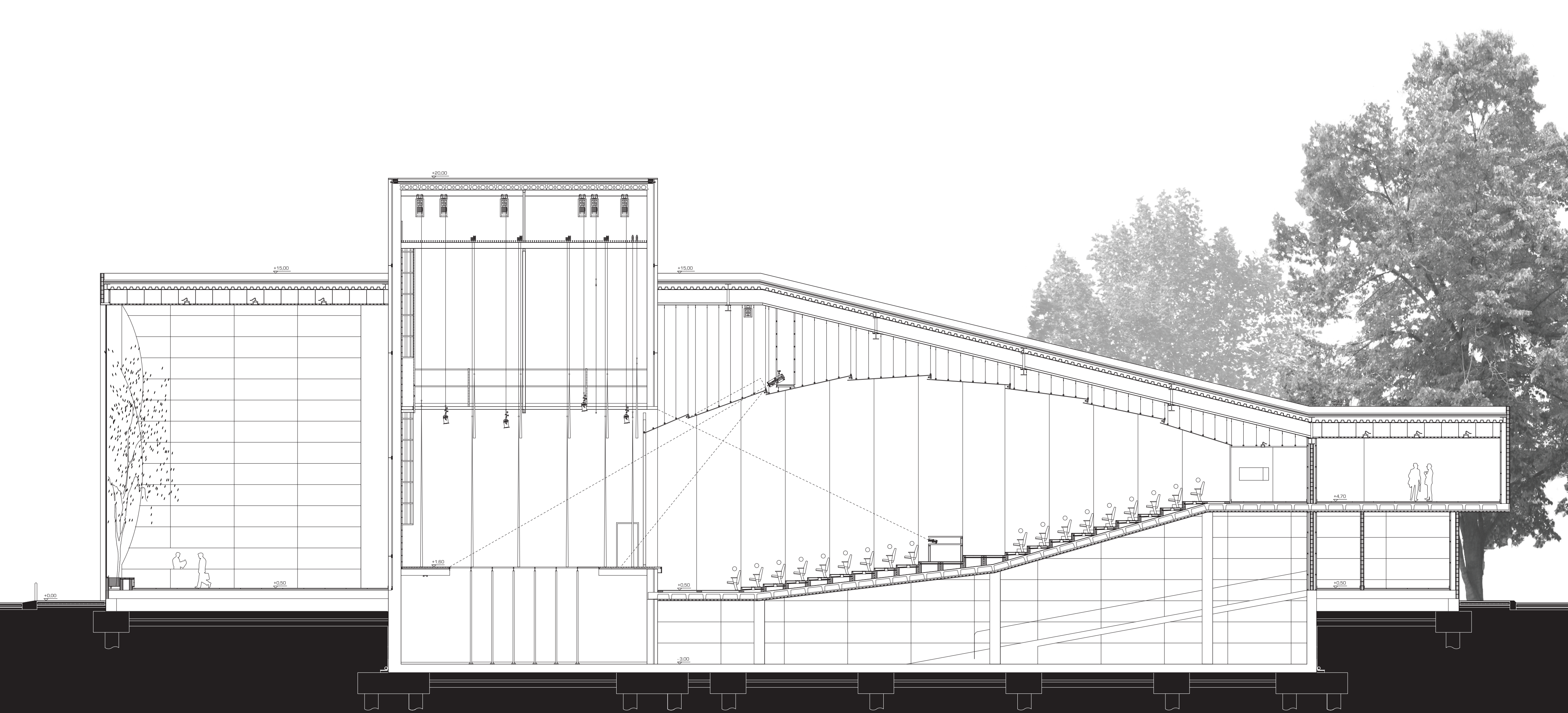
Sección Longitudinal Constructiva. Escala 0 5 15 m
