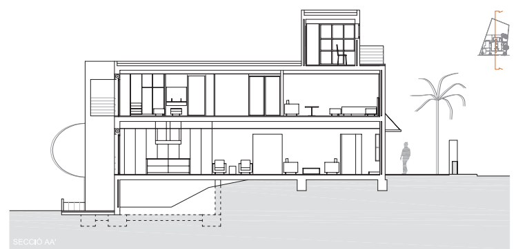
SECCIÓ AA'
