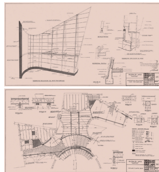
Nártex de la iglesia. Perspectiva (realización del muro prefabricado), y planta del forjado de planta baja (Vitrino Histórico del Colegio Territorial de Arquitectos de Alicante)
