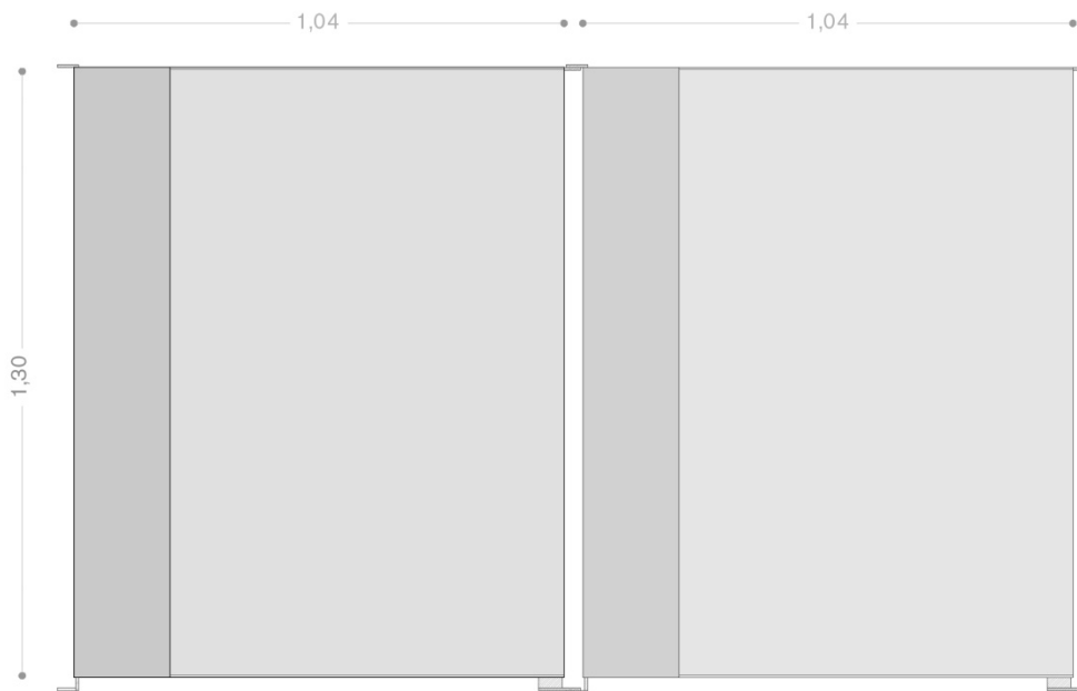
Alzado elemento superior 1,30 x 1,04m
